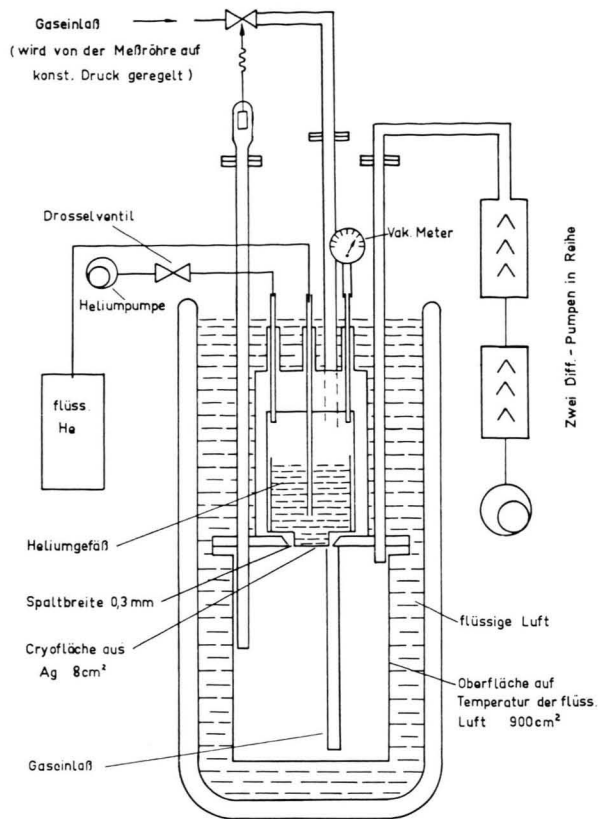
Abb. 1. Versuchsaufbau der Kryopumpe.
